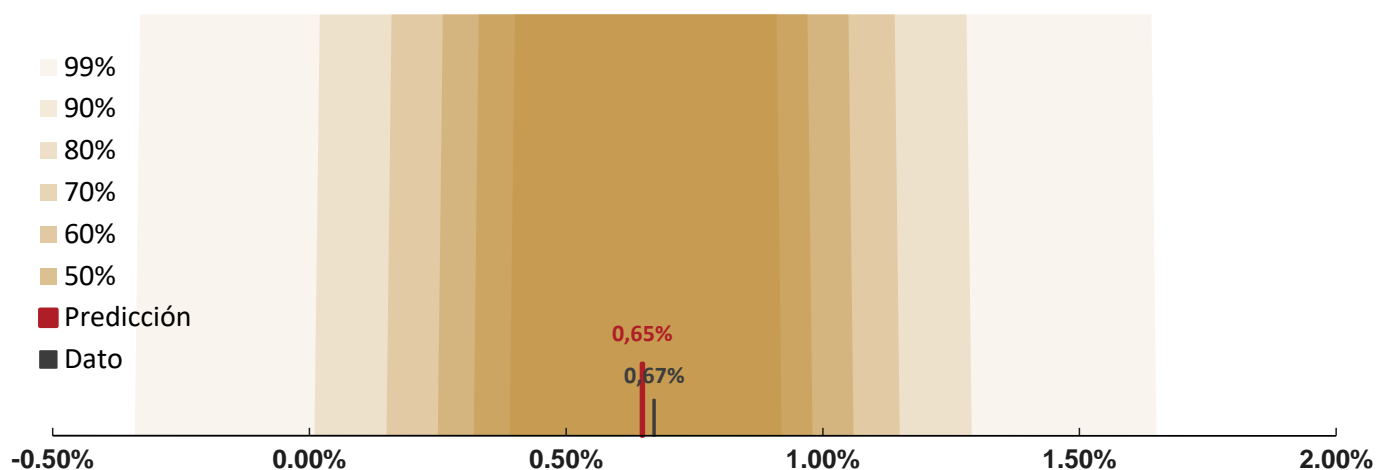
Gráfico: Predicción puntual e intervalos de probabilidad para la inflación de junio, y dato observado
