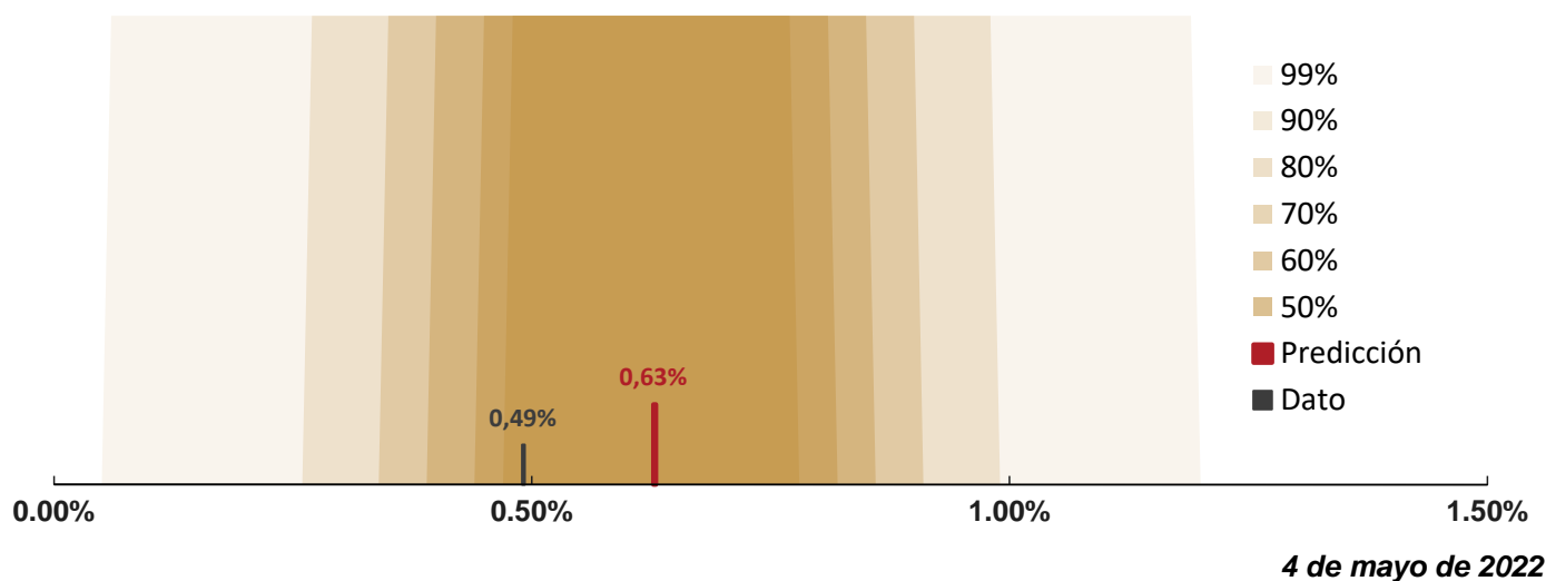
Gráfico: Predicción puntual e intervalos de probabilidad para la inflación de abril, y dato observado
